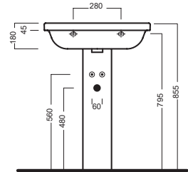
colonna_pedestal
