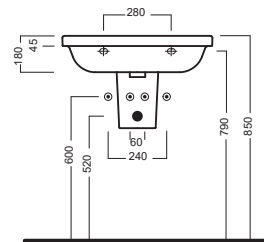
semicolonna_siphon cover
